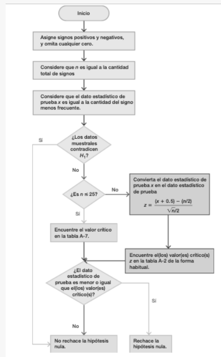
Procedimiento de la Prueba de Signo.
